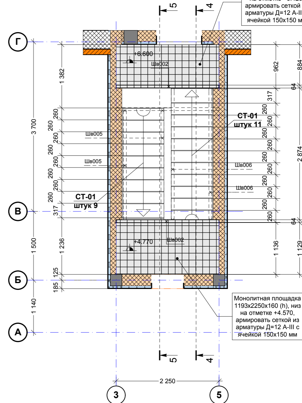
Спецификация изделий и материалов к чертежам 40-Схема лестничной клетки
