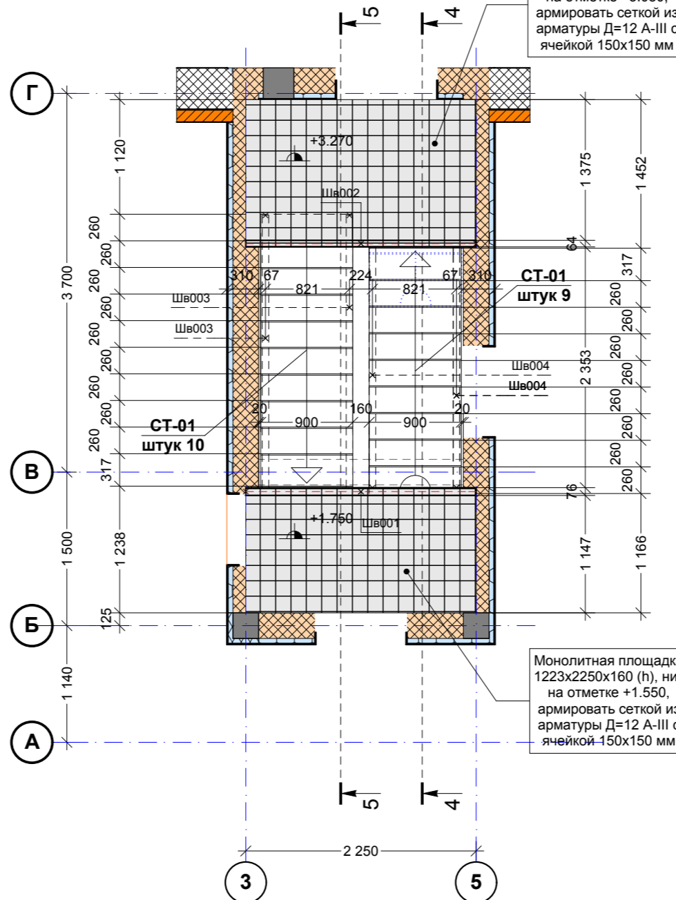
План на отметке +3.300 (сечение 2-2 - лист 41)
