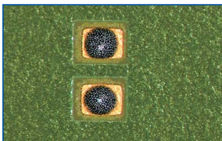
Рис. 4. Слой нанесенной пасты на контактные площадки компонента 0201
